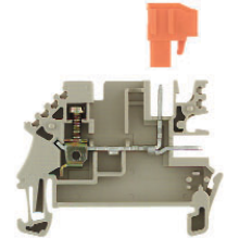
WDU 2.5/BLZ R 7.62
