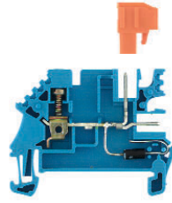
WDU 1.5/BLZ/R 5.08
