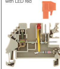
WDU 1.5/BLZ/LD 5.08
