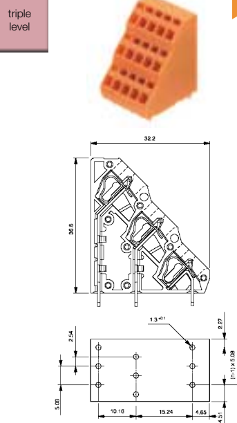
LM3RZF 5.08/135
