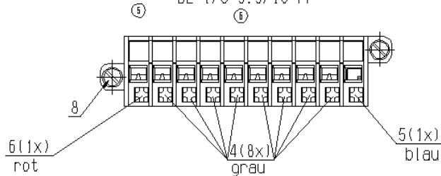
Ausführungsvorschrift Frontplatte
