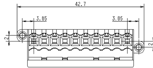
Ansicht X
