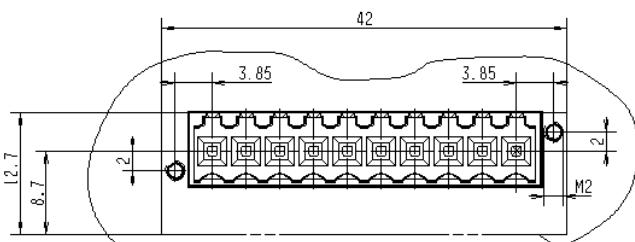
Ausführungsvorschrift Frontplatte
