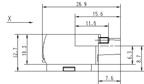
Ansicht X
