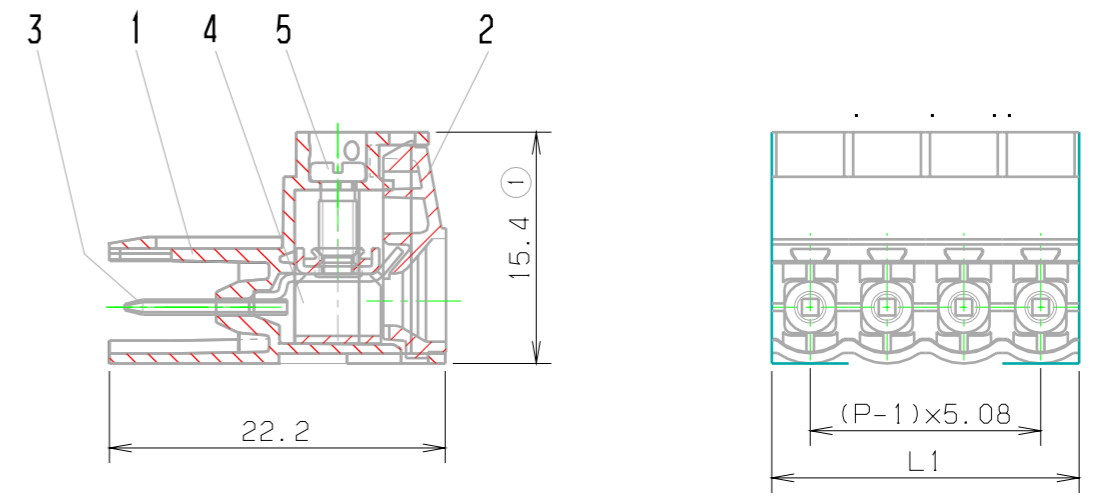
Ausführung: SLS 5.08/2..24 ohne jeglichen Schwalbenschwanz
