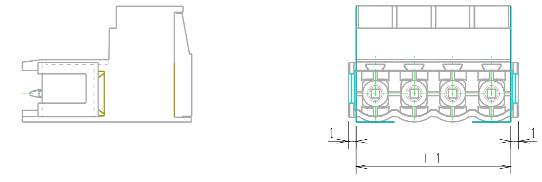
Ausführung: SLS 5.08/2..24B mit seitlichen Schwalbenschwanz für BBl. ...
