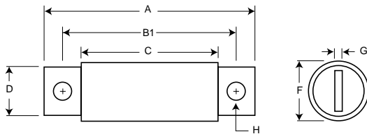
Fig. 1: 1-30 & 450-1000 Amp Range
