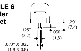
STYLE 7 Wire Wrap
