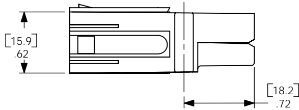
45° HOOD
